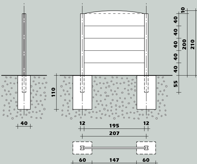
Abmessungen „Standard L“ H = 2,10 m
